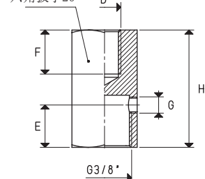
六角扳手20
