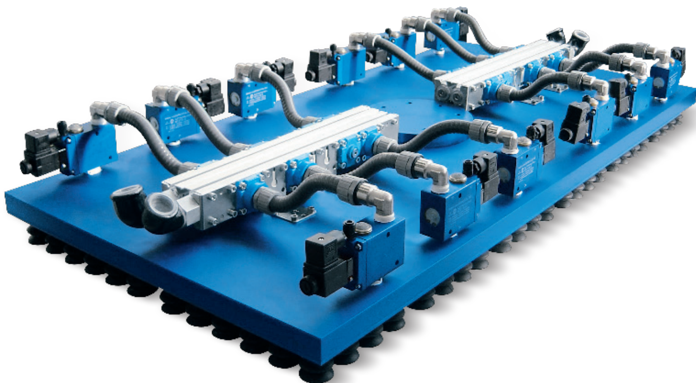
mm 620x1240 配12个独立蓄能室 - SO 62 127 2V
