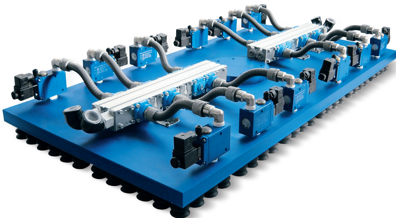
mm 620x1240 配12个独立蓄能室 - S0 62 127 2V
