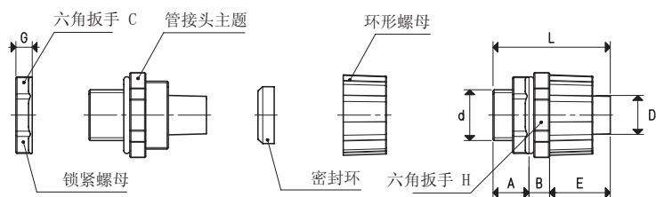
RTPR管接头
