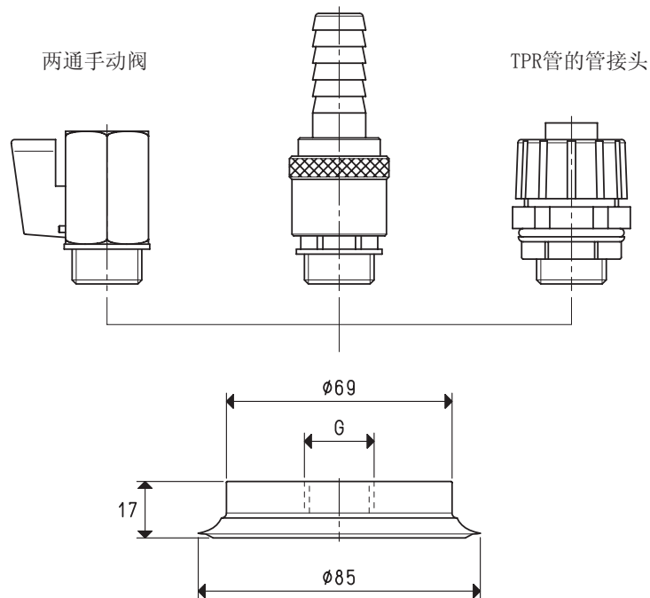
快插式管接头
