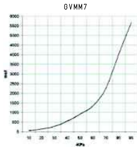
不同真空度(-Kpa)下所需的抽气时间 (ms/l=s/m³)
