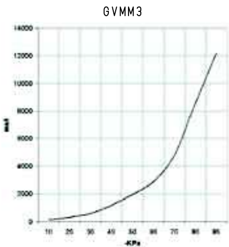
不同真空度(-Kpa)下所需的抽气时间 (ms/l=s/m³)
