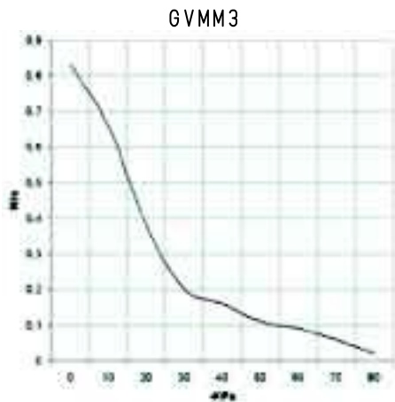
在不同真空度 (-Kpa) 下的抽气量 (NI/S)
