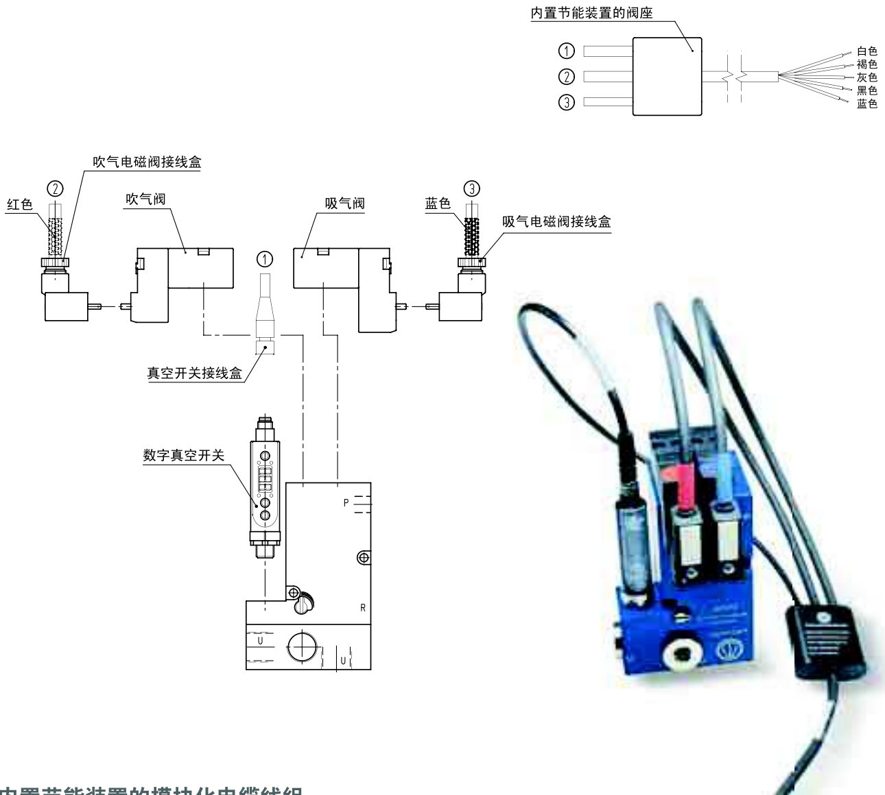
内置节能装置的模块化电缆线组
