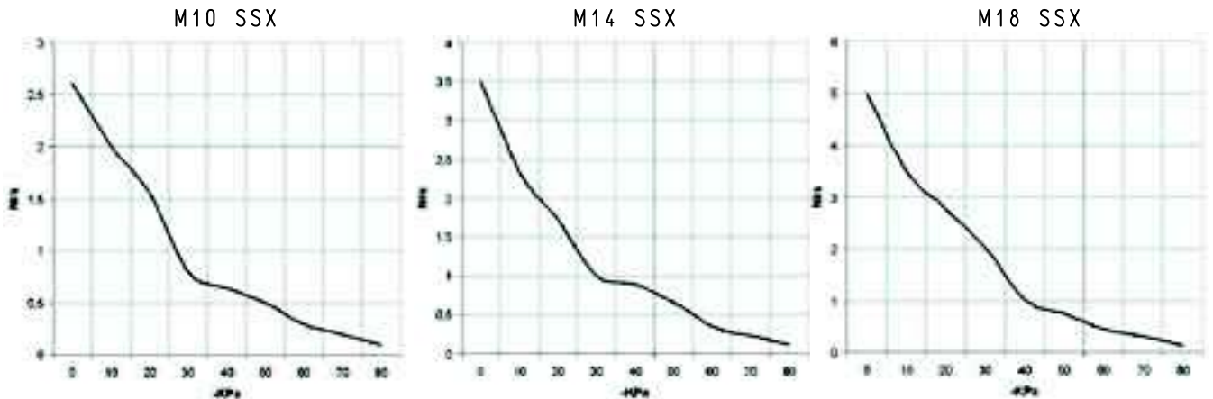
在不同真空度 (-Kpa) 下的抽气量 (NI/S)
