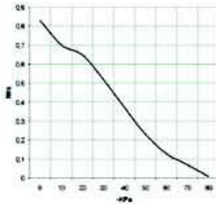
在不同真空度 (-Kpa) 下的抽气量 (NI/S)
