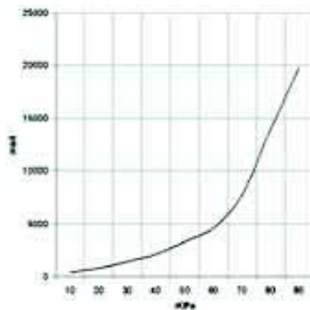
不同真空度(-Kpa)下所需的抽气时间 (ms/l=s/m³)
