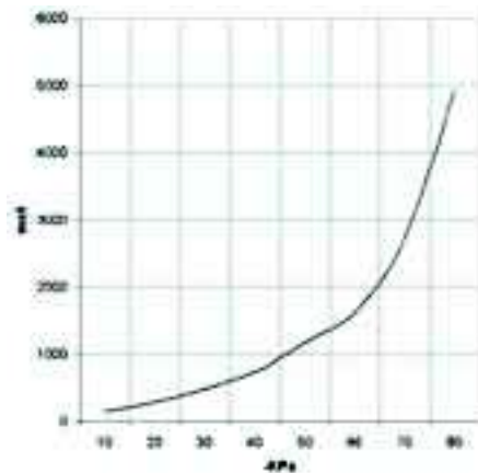
不同真空度(-Kpa)下所需的抽气时间 (ms/l=s/m 3 )
